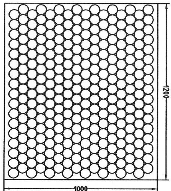
Packschema: Querverpackt 14/14 x 20
